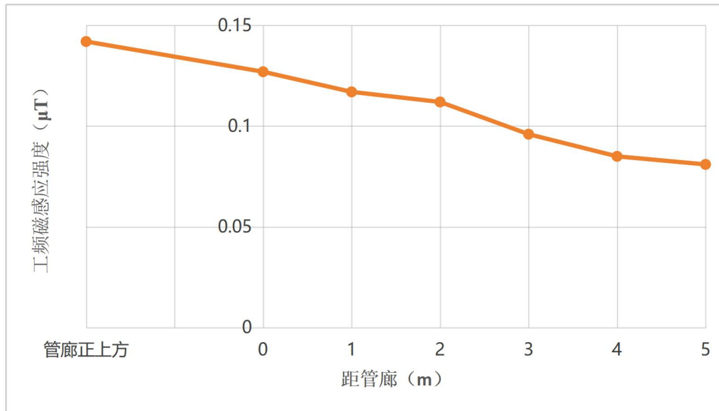
图3-2 类比断面工频磁感应强度的变化趋势图
