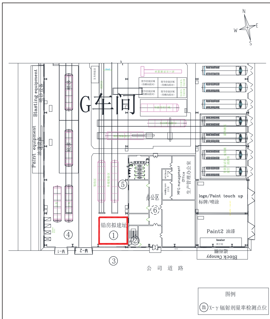
图 8-5 公司 IMC 探伤铅房拟搬迁场址及周围辐射环境现状检测点位示意图
