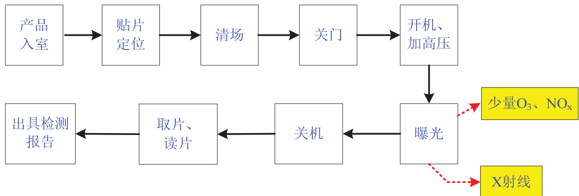
图 9-5 X 射线探伤机开展固定探伤工作流程及产污环节分析示意图
