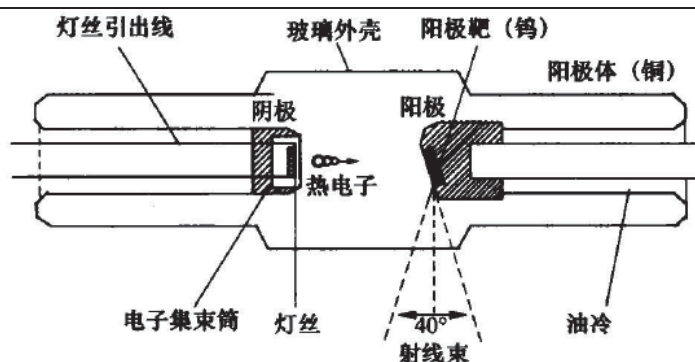
图 9-3 X 射线探伤机结构示意图
